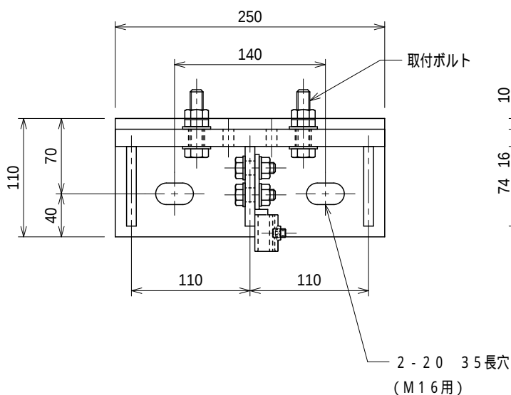
架台リブ詳細図 S = 1 : 4
