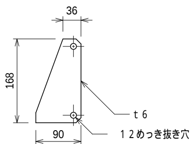
架台リブ詳細図
