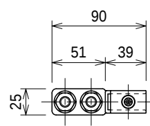
Z端子 片側付 (品番：S7141)
