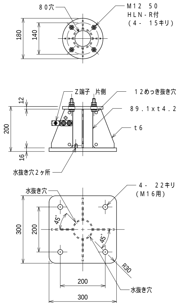
架台詳細図
